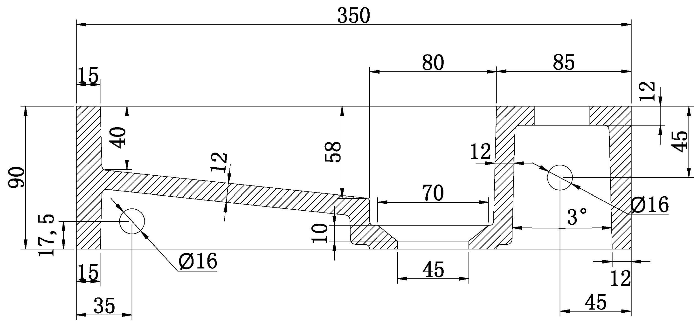
A-A
